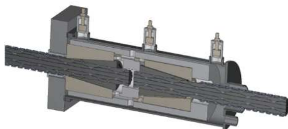
例 モノグリップ型カブラー
