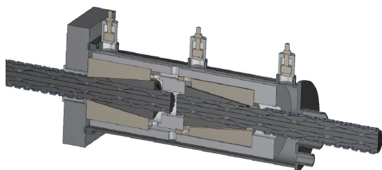
例 モノグリップ型カプラー
