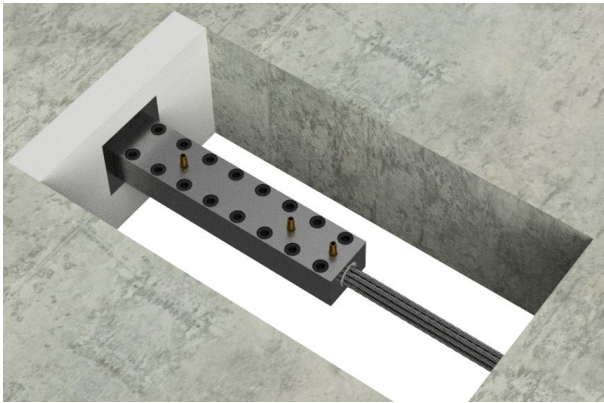
膨張材式中間定着装置
