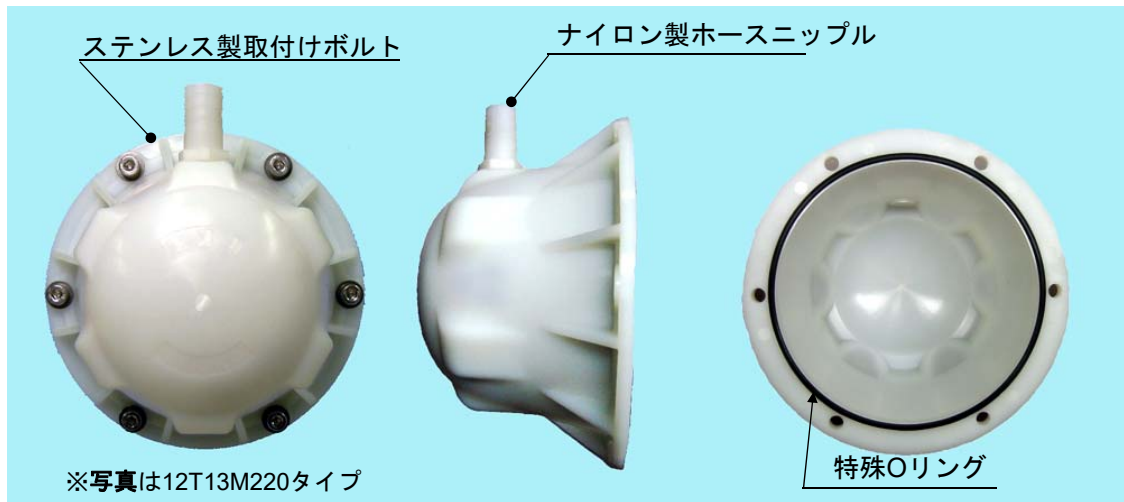
樹脂製グラウトキャップ
